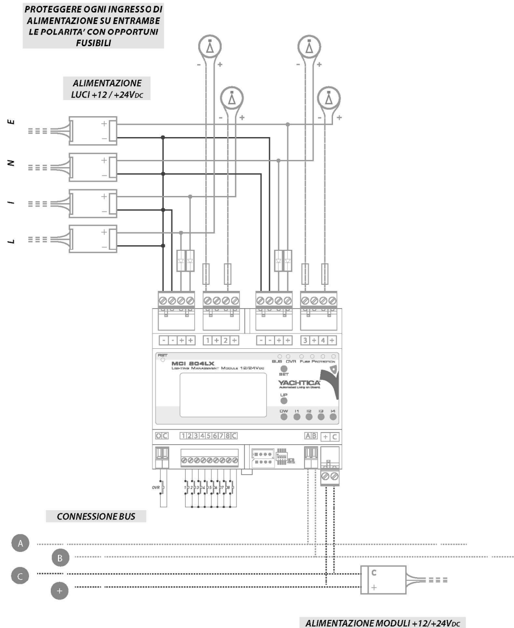
SCHEMA 3: Collegamento positivo diretto con alimentatori indipendenti
