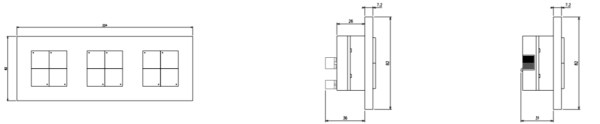
Vista frontale
